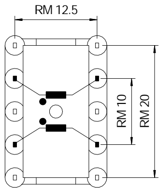
Ansicht von unten (Lötseite)
