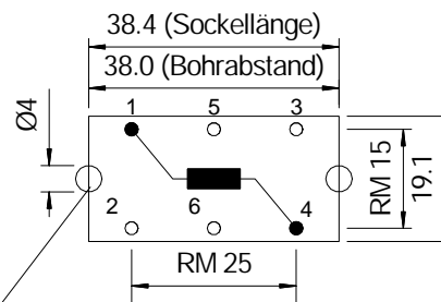
Ansicht von unten (Lötseite)
